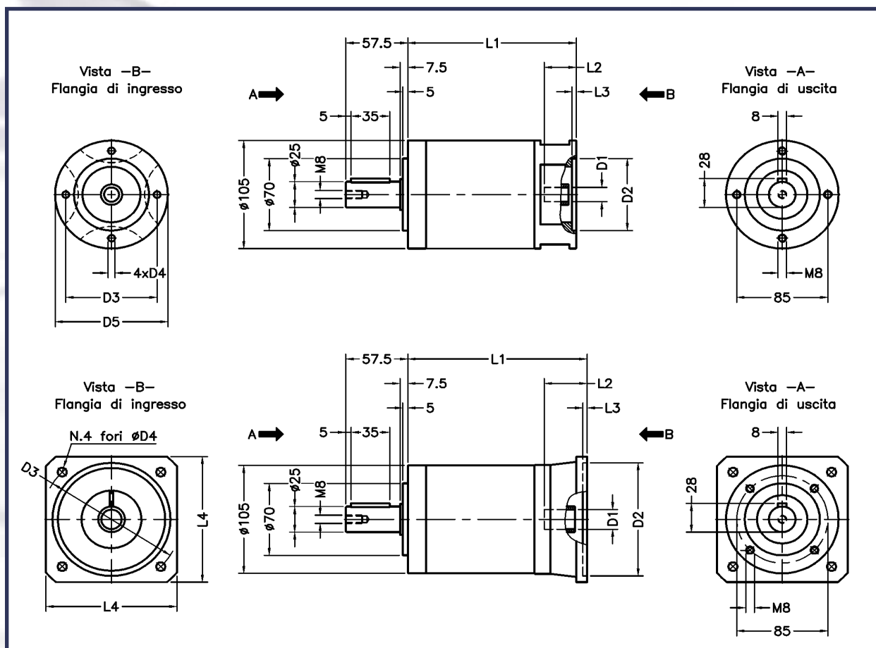
DIMENSIONI ALBERO IN INGRESSO - INPUT SHAFT DIMENSIONS
